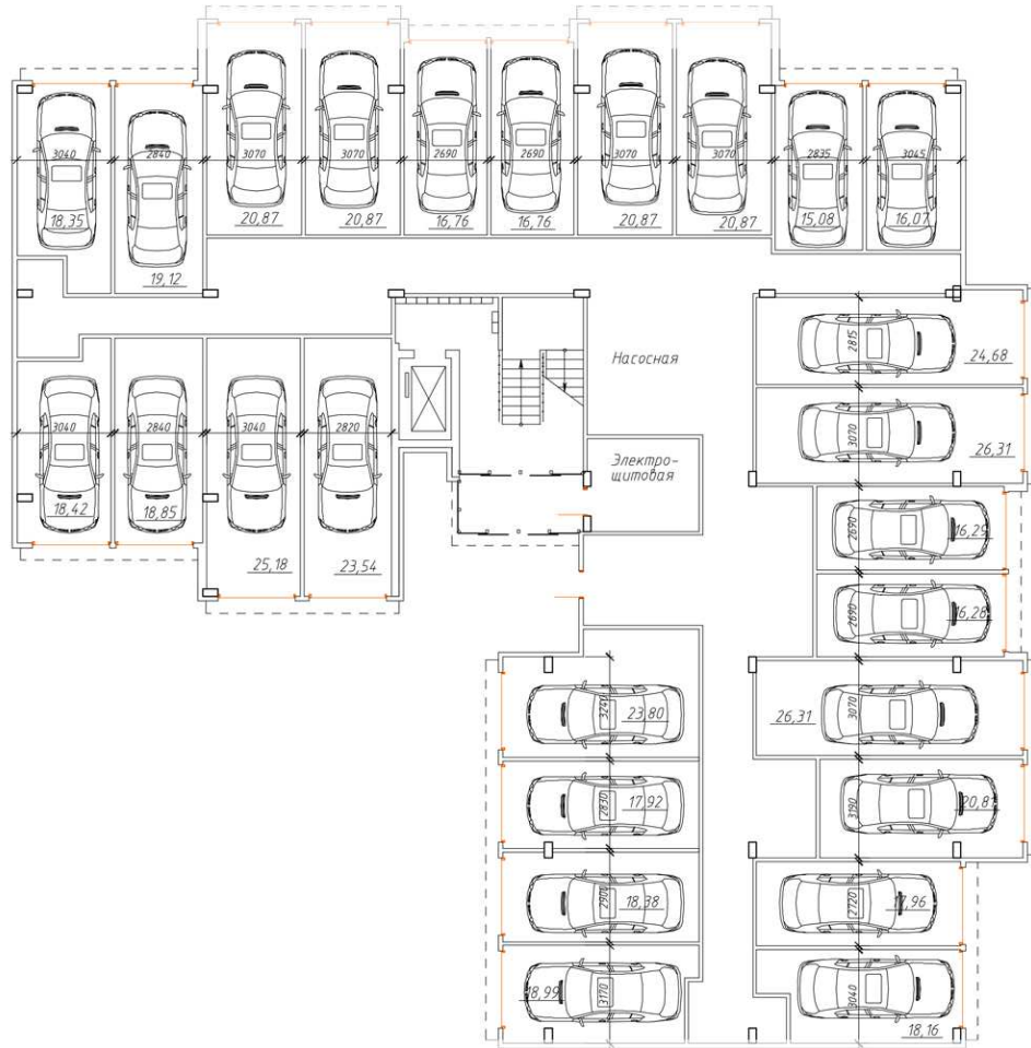
План 1-ого этажа
